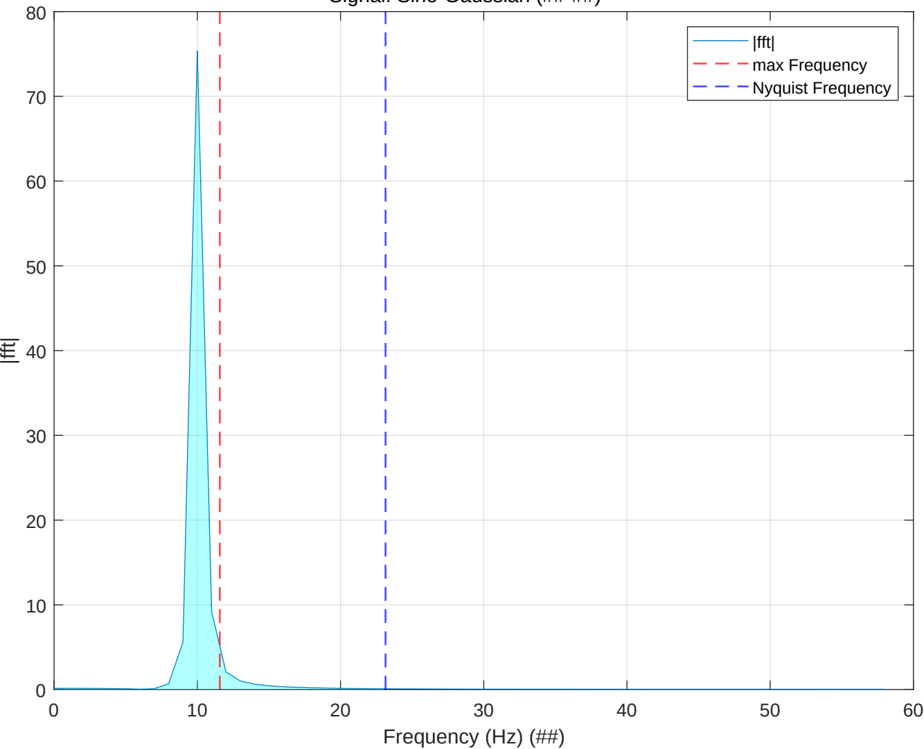
Signal: Sine-Gaussian (##-##)
